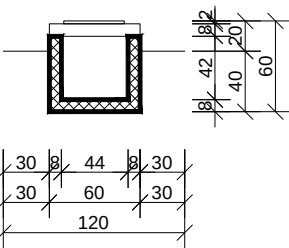
POPREČNI PRESJEK
