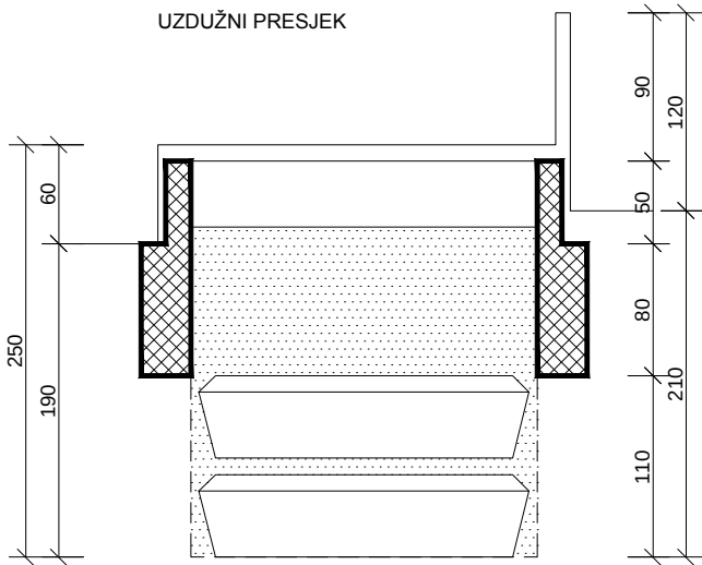
UZDUŽNI PRESJEK
